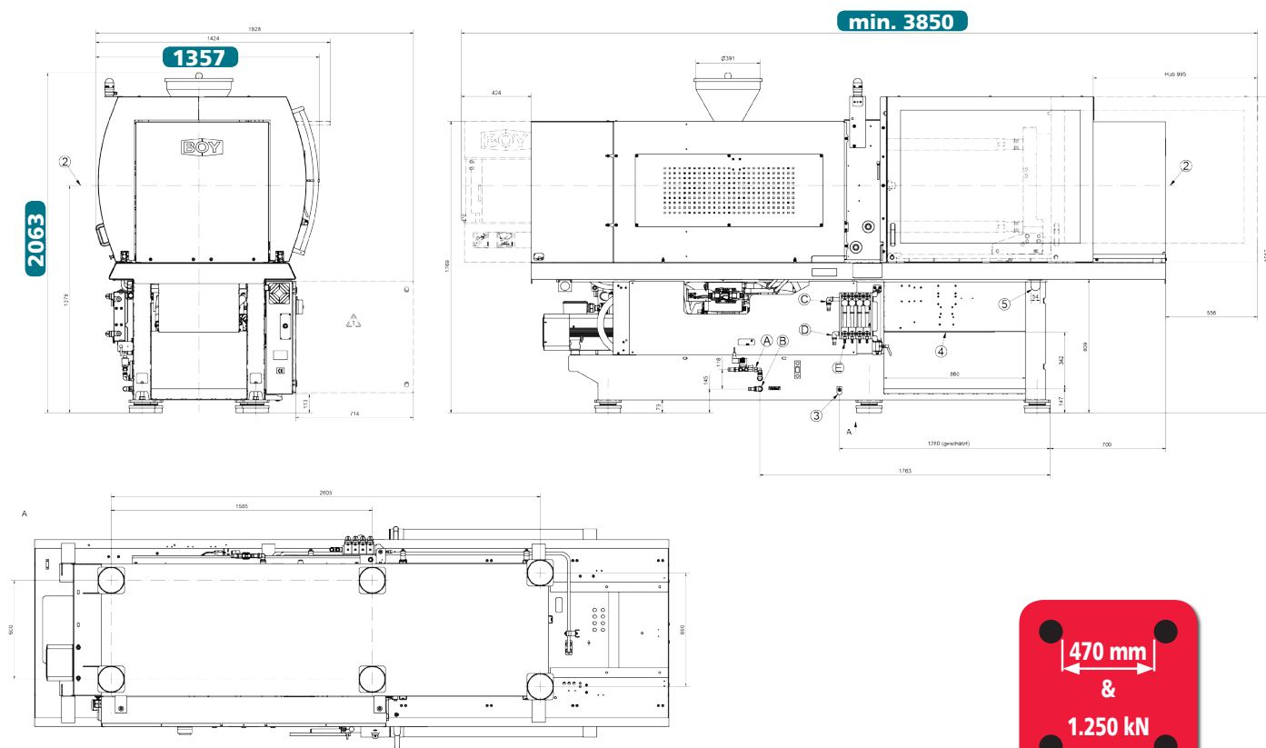
BOY 125 E
